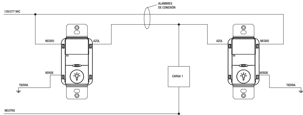
DIAGRAMA DE CABLEADO DE 3 VÍAS: LAS LUCES SE APAGARÁN, CUANDO LA UNIDAD QUE SE ENCENDIÓ ÚLTIMAMENTE Y/O DETECTÓ MOVIMIENTO ÚLTIMAMENTE FINALIZA SU RETARDO DE TIEMPO.
