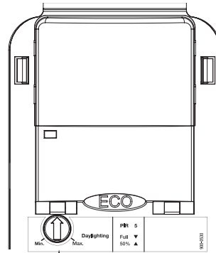
Ajuste del nivel del sensor de luz del día
