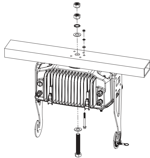
12b Local Pendant Mount
