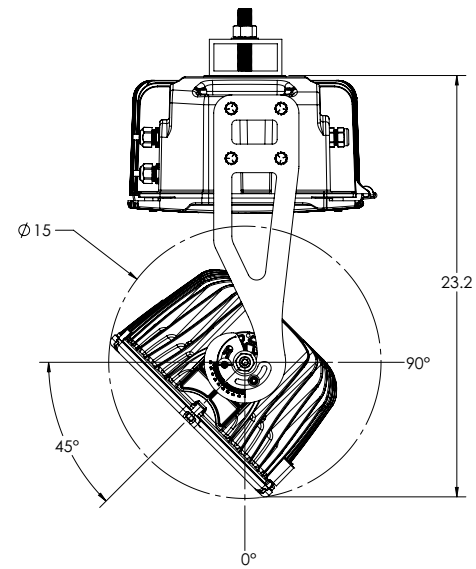
4a Pendant Mount
