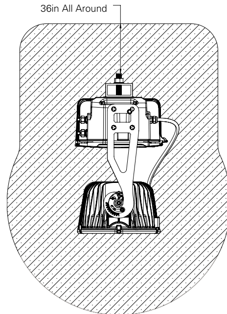
1b Pendant Mount
