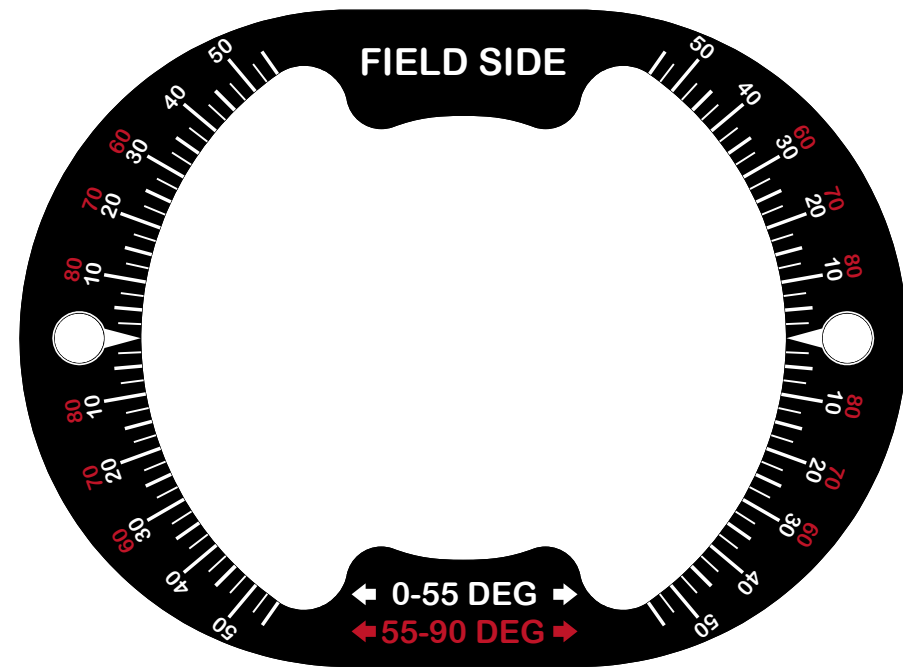
12b Local Pendant Mount
